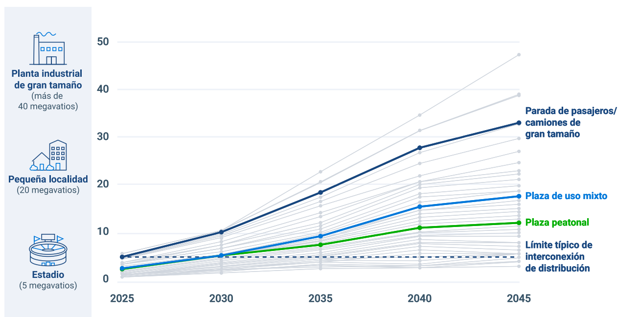
Fig. 03 – Capacidad de carga del proyecto para 71 emplazamientos en carreteras del noreste (megavatios de potencia para satisfacer la demanda máxima anual, a lo largo del tiempo)
